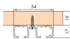
B mit Drehriegel (nicht für Hartholz/MDF) with swivel lug (not for hard wood/MDF) avec verrou (pas pour bois dur/MDF)
